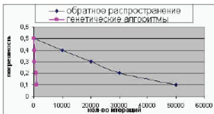
Рис. 5. Сравнение результатов работы генетических алгоритмов и алгоритма обратного распространения (первый случай)
