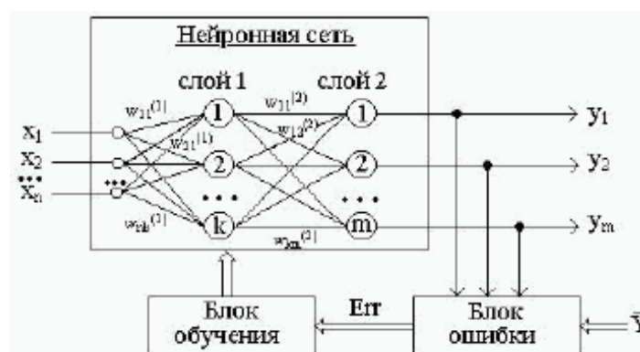
Рис. 1. Обучение «с учителем» многослойной нейронной сети
