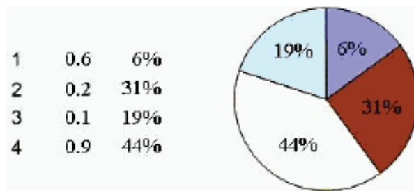
Рис. 2. Оператор селекции типа колеса рулетки с секторами пропорциональными функции приспособленности
