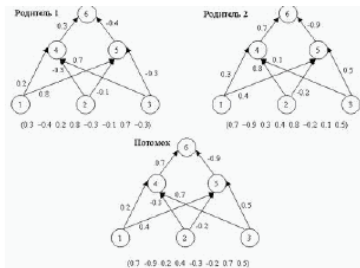
Рис. 3. Оператор скрещивания
