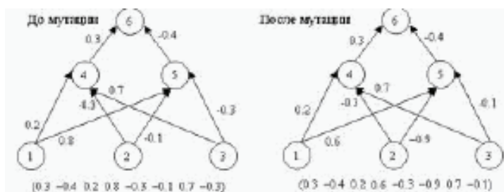
Рис. 4. Оператор мутации
